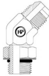
JICM X UNOM 45° ELBOW (M X M)
