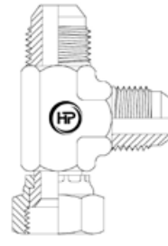
JICM X JICF X JICM RUN TEE
