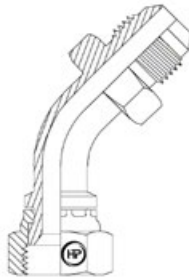
JICM X JICF 45° BEND (M X F)
