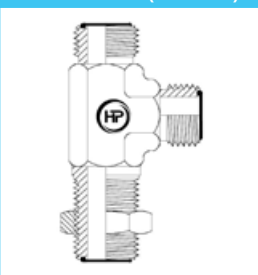
ORFSM X ORFSM(BH) X ORFSM TEE BULKHEAD (M X M X M)
