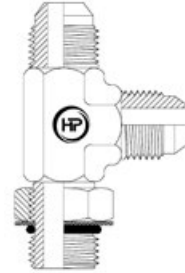
JICM X UNOM X JICM RUN TEE
