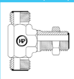
ORFSM X ORFSM X ORFSM(BH) TEE BULKHEAD (M X M X M)
