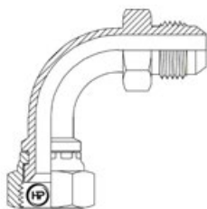
JICM X JICF 90° BEND (M X FS)
