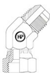
JICM X JICF 45° ELBOW (M X F)
