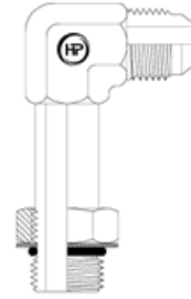
JICM X UNOM EXT. 90° ELBOW (M X M)
