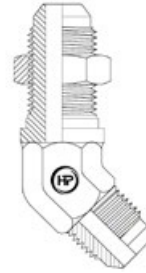
JICM X JICM 45° BULKHEAD
