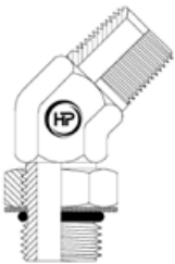
BSPTM X UNOM 45° ELBOW (M X M)
