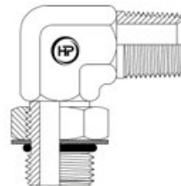
BSPTM X UNOM 90° ELBOW (M X M)
