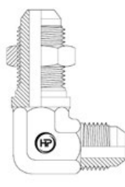
JICM X JICM 90° BULKHEAD
