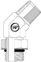
BSPTM X UNOM 45° ELBOW (M X M)
