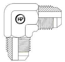
JICM X JICM 90° ELBOW (M X M)
