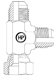
JICM X JICF X JICM RUN TEE
